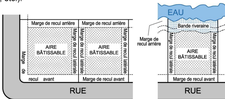
Croquis 2.1 Aire bâtissable et marges de recul d'un terrain pour diverses situations
