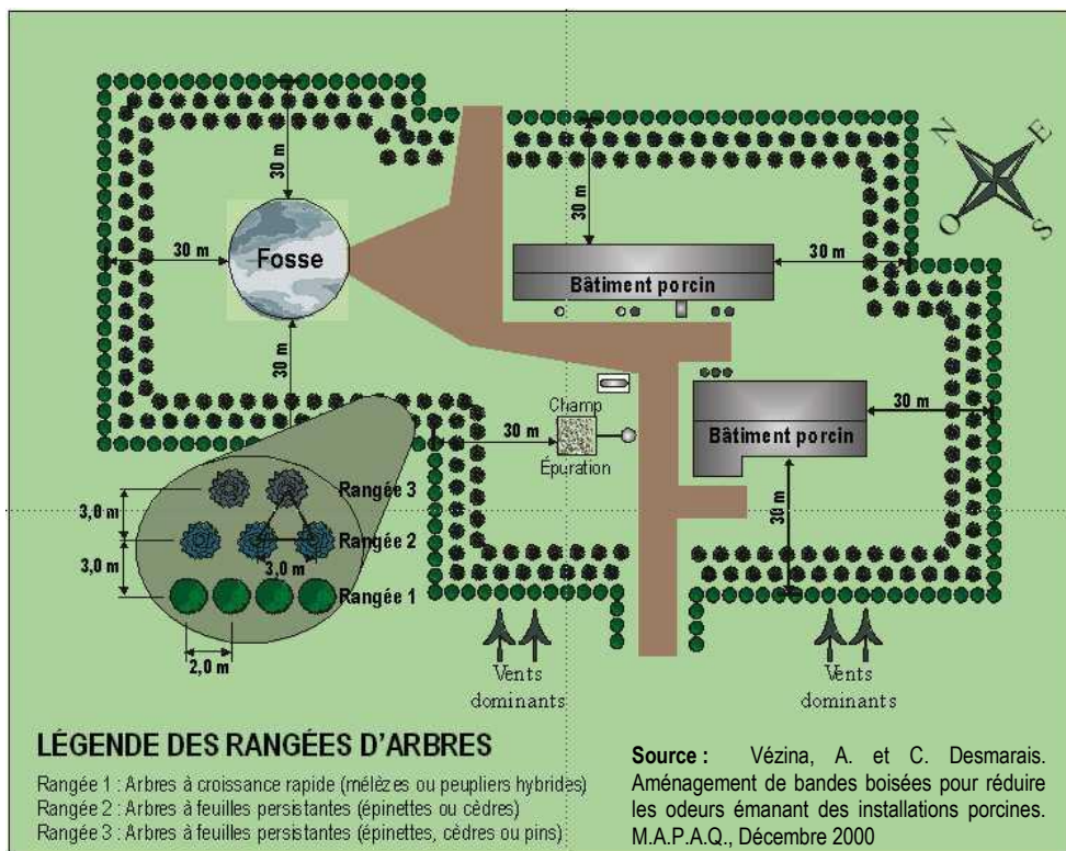
Croquis 15.1 : Schéma illustrant l'aménagement d'une haie brise-vent autour d'une installation d'élevage
